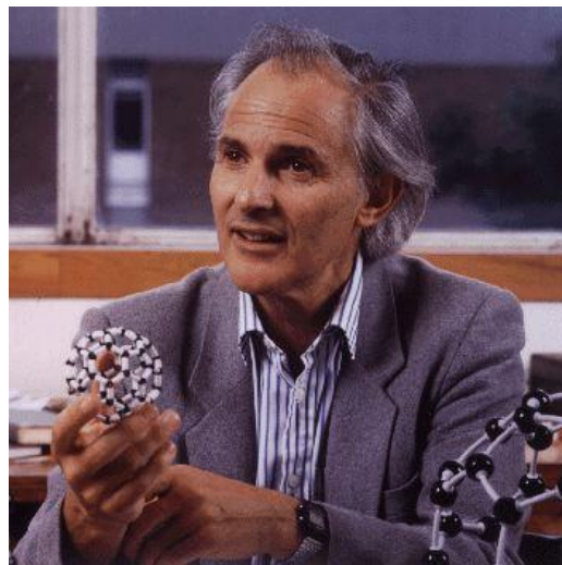
H.W. Kroto
