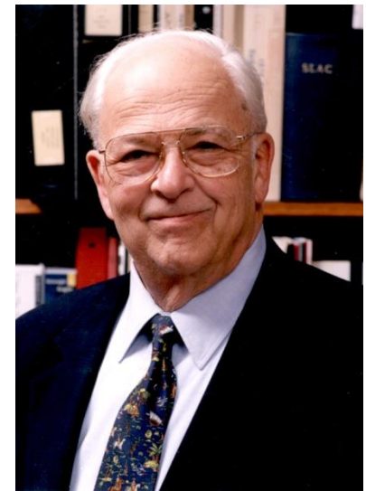
Burton Richter
